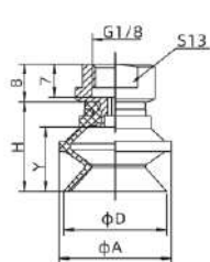
SZB17...20□-G1F
