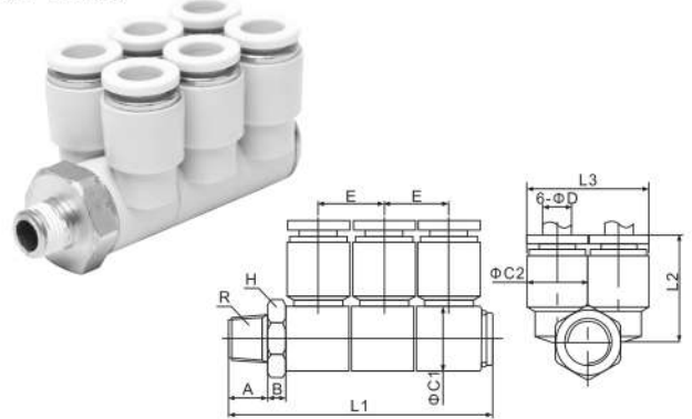
KQ2ZT 系列-3个双管万向弯头 KQ2ZT Series
