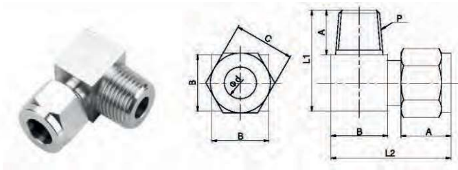
Серия YZ2-2 — Угловой с наружной резьбой
