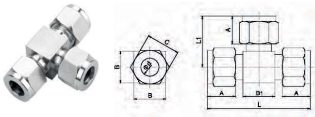
Серия YZ2-5 — Проходной тройник
