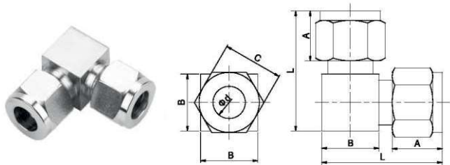
Серия YZ2-4 — Угловой патрубок
