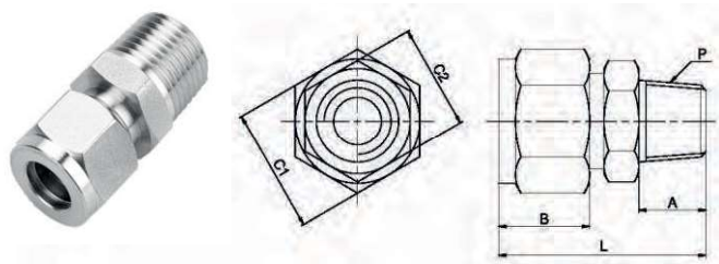
Серия YZ2-1 — Прямой с наружной резьбой
