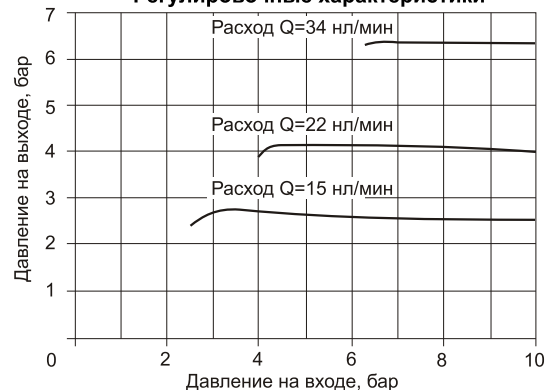
Регулировочные характеристики
