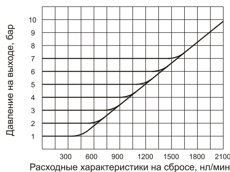
Регулировочные характеристики (17312A.C)
