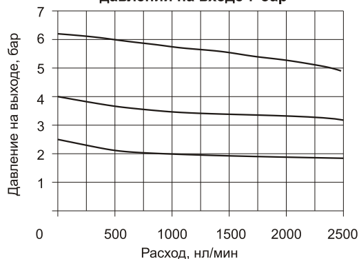
Регулировочные характеристики
