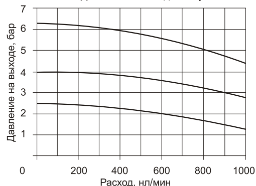
Регулировочные характеристики
