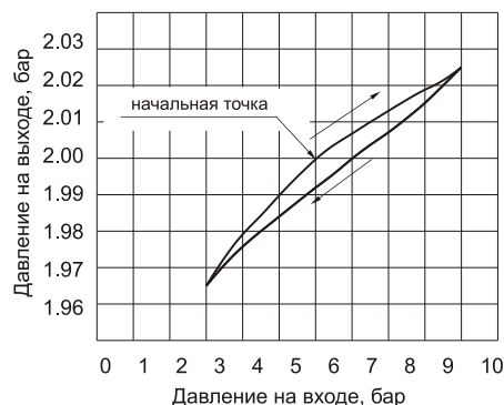
Регулировочные характеристики (17312A.C)
