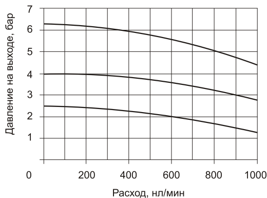
Расходные характеристики при давление на входе 7 бар
