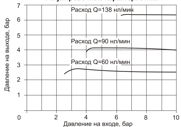
Регулировочные характеристики
