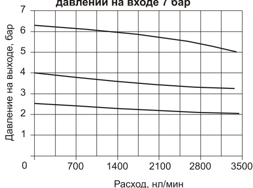
Регулировочные характеристики
