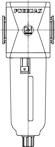
Размер 1-2-3 Кожух или колба из металла
